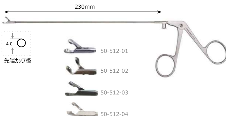
S&T 喉頭検査用マイクロ鉗子 (ラウンドカップ) (mm)
