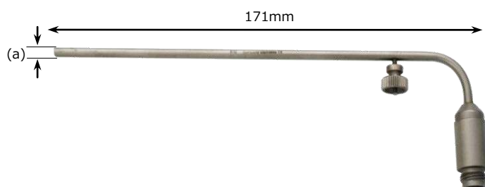
S&T ライトキャリア (mm)
