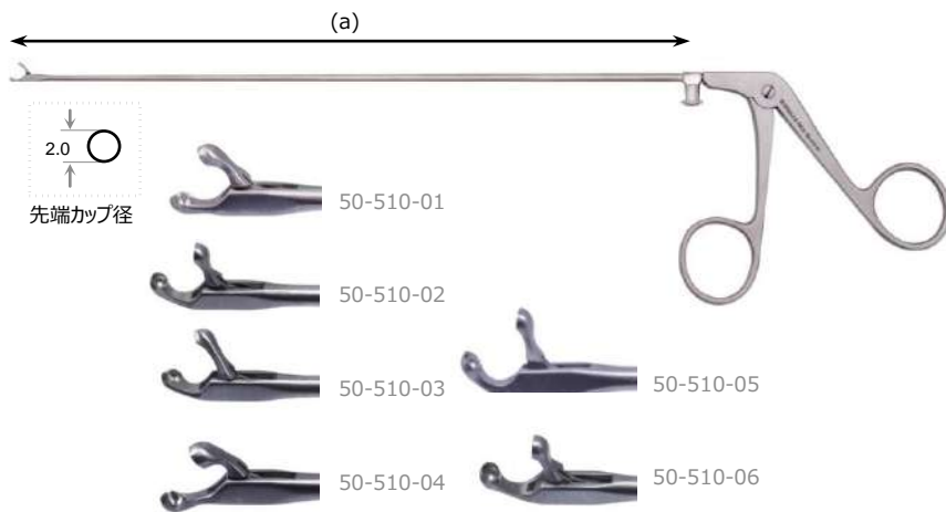
S&T 喉頭検査用マイクロ鉗子 (ラウンドカップ) (mm)
